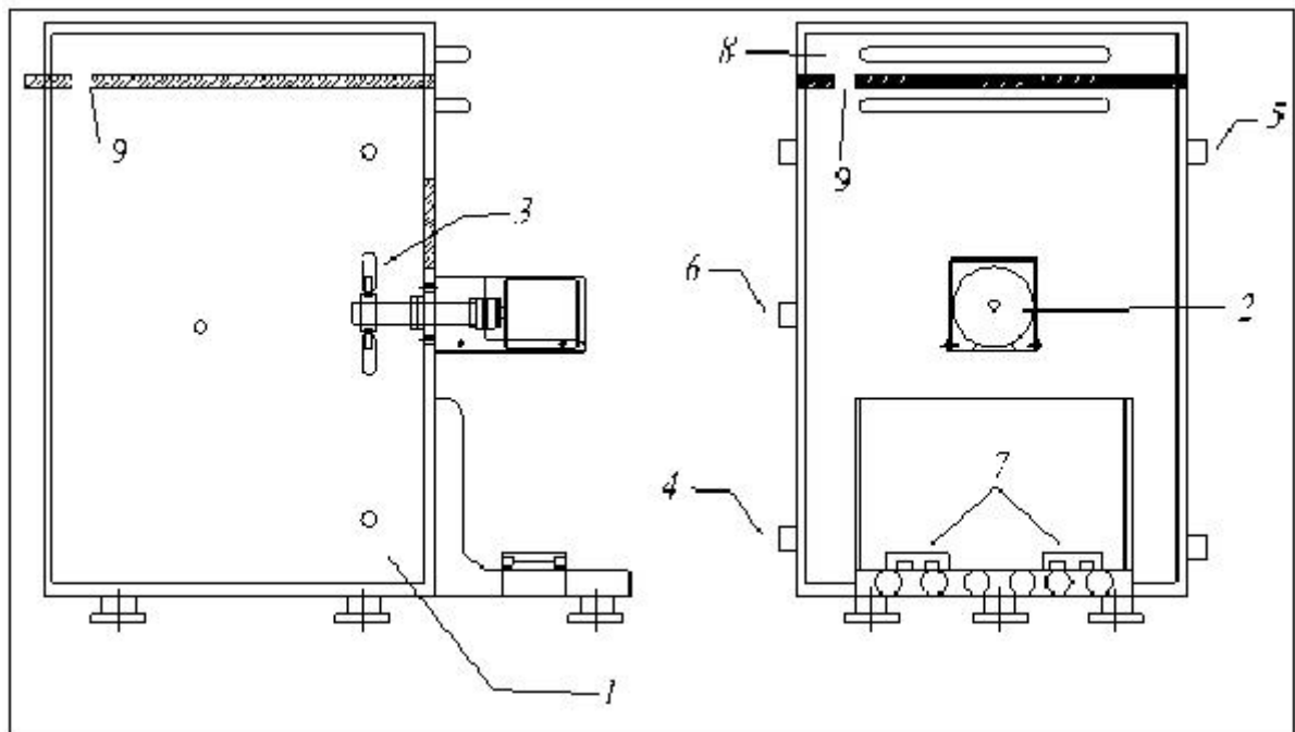
Hình 4a: Phòng thử nổ loại 1 ngăn
